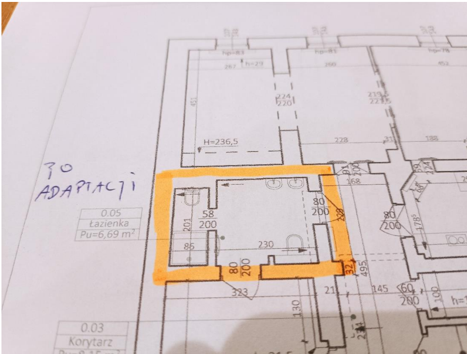
Rysunek 1 – Rzut łazienki po adaptacji
